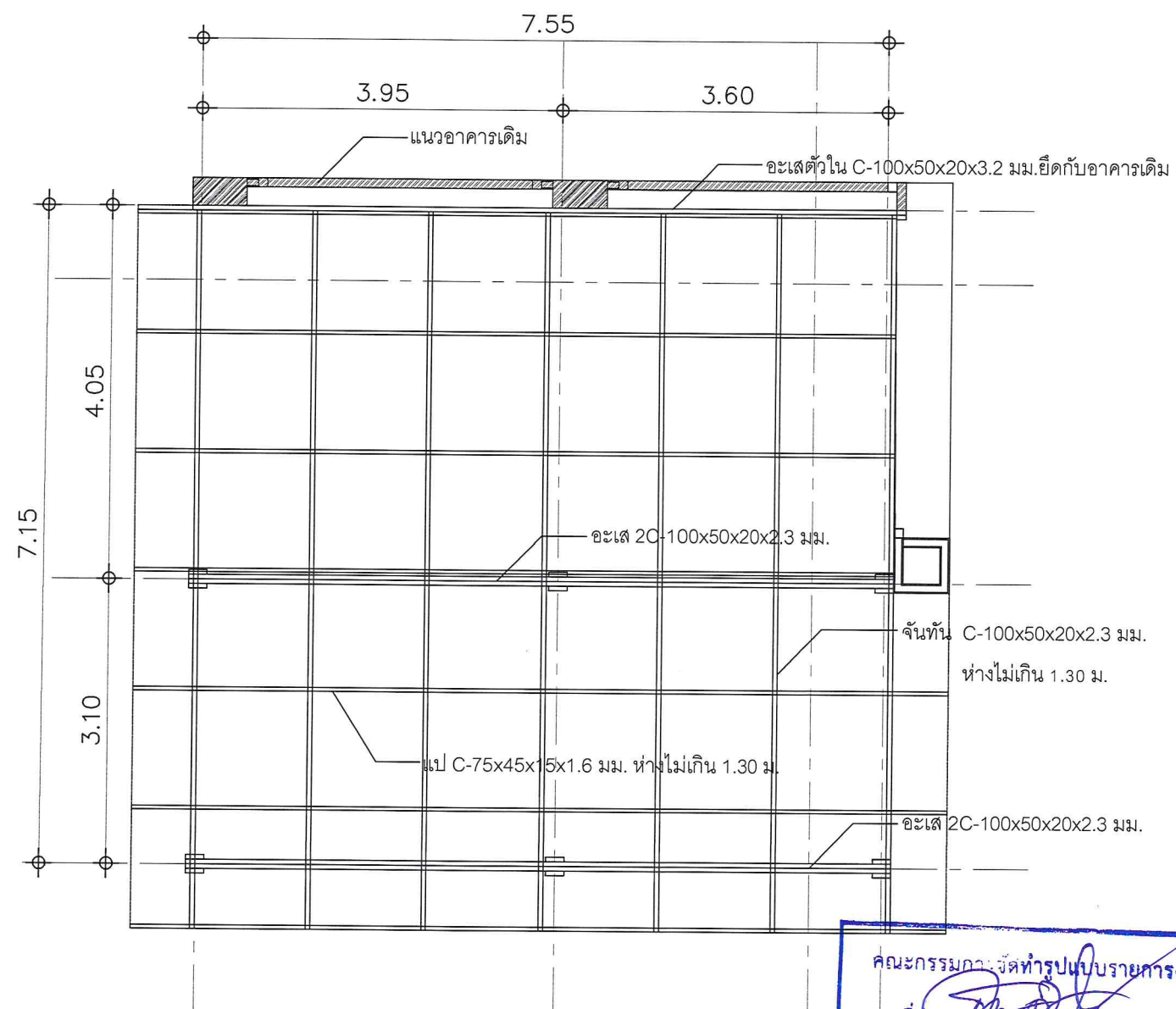
แปลนโครงหลังคา ต่อเติมด้านหน้าอาคาร อบต.ทับใต้ 2 scale 1:75
