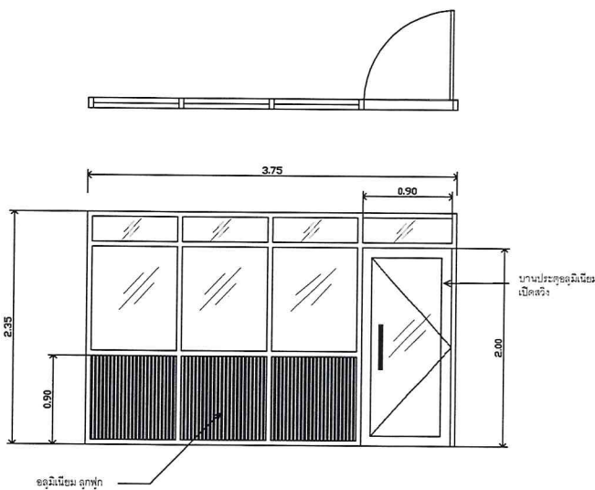
แบบขยายผนังอลูมิเนียม พร้อมประตู ต่อเติมภายในอาคาร อบต.ทับใต้ 2 scale 1:25
