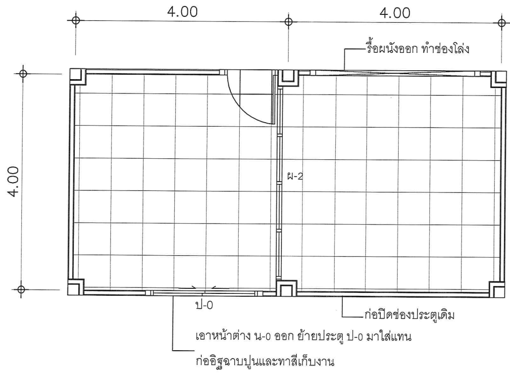
แบบแปลน งานปรับปรุงภายใน อบต.ทับใต้ อาคาร 2
