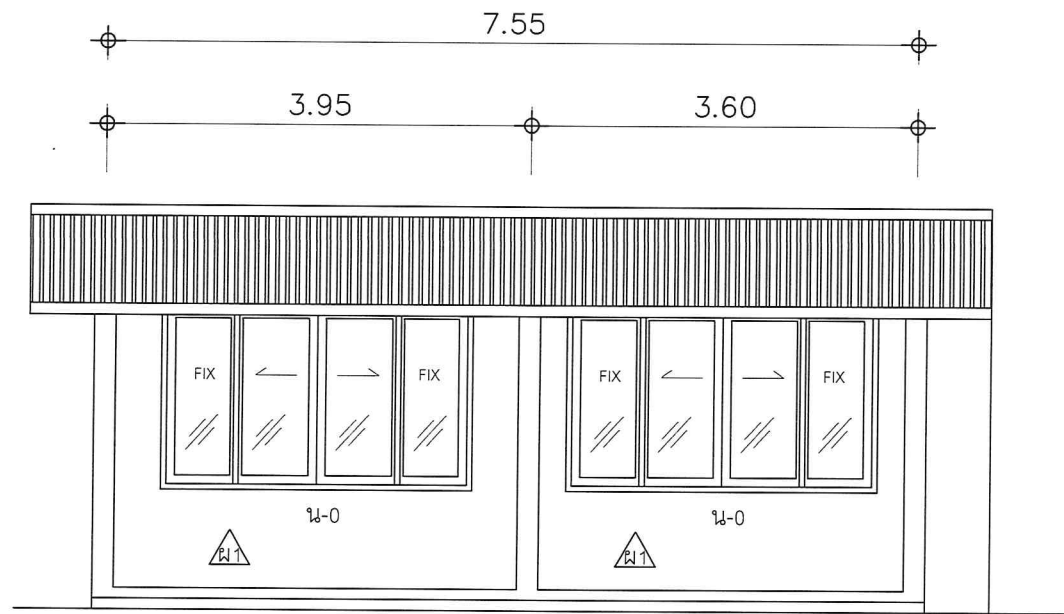
รูปด้านหน้าต่อเติมอาคาร อบต.ทับใต้ 2 scale 1:75
