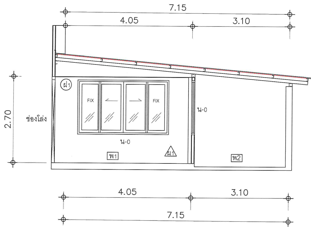
รูปตัด 1-1 ต่อเติมอาคาร อบต.ทับใต้ 2 scale 1:75
