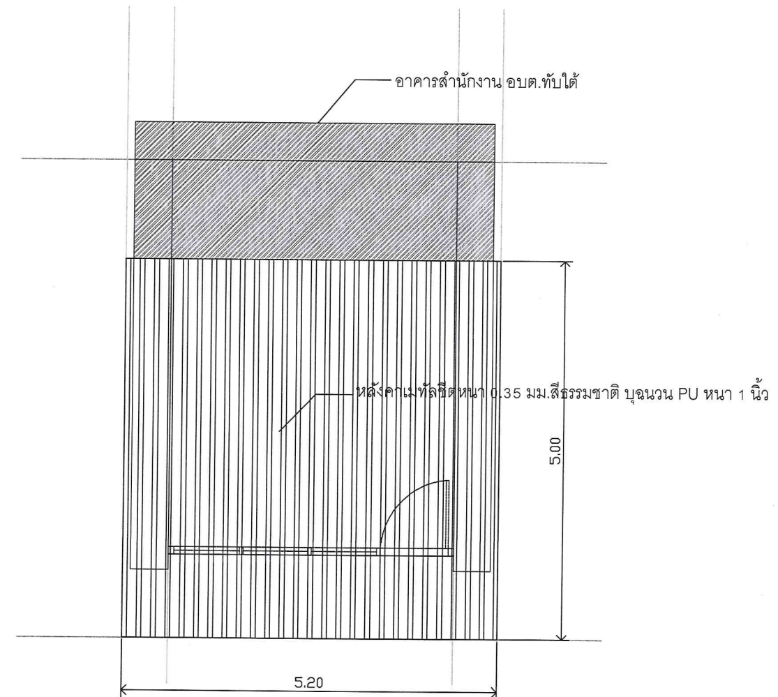
แปลนหลังคา ต่อเติมด้านหลัง อาคารสำนักงาน อบต.ทับใต้ scale 1:75
