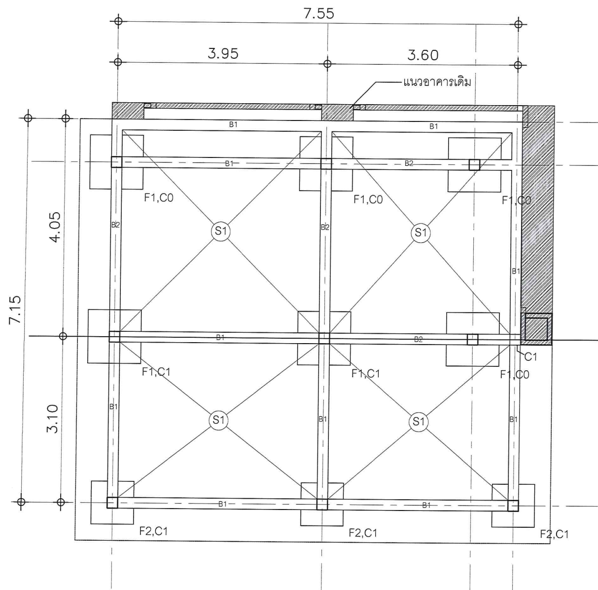
แปลนโครงสร้าง สานราก เสาคาน พื้น ต่อเติมด้านหน้าอาคาร อบต.ทับใต้ 2 scale 1:75
