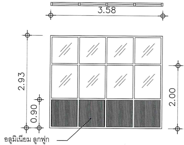
แบบขยายผนัง ผ-2 งานปรับปรุง อบต.ทับใต้ อาคาร 2
